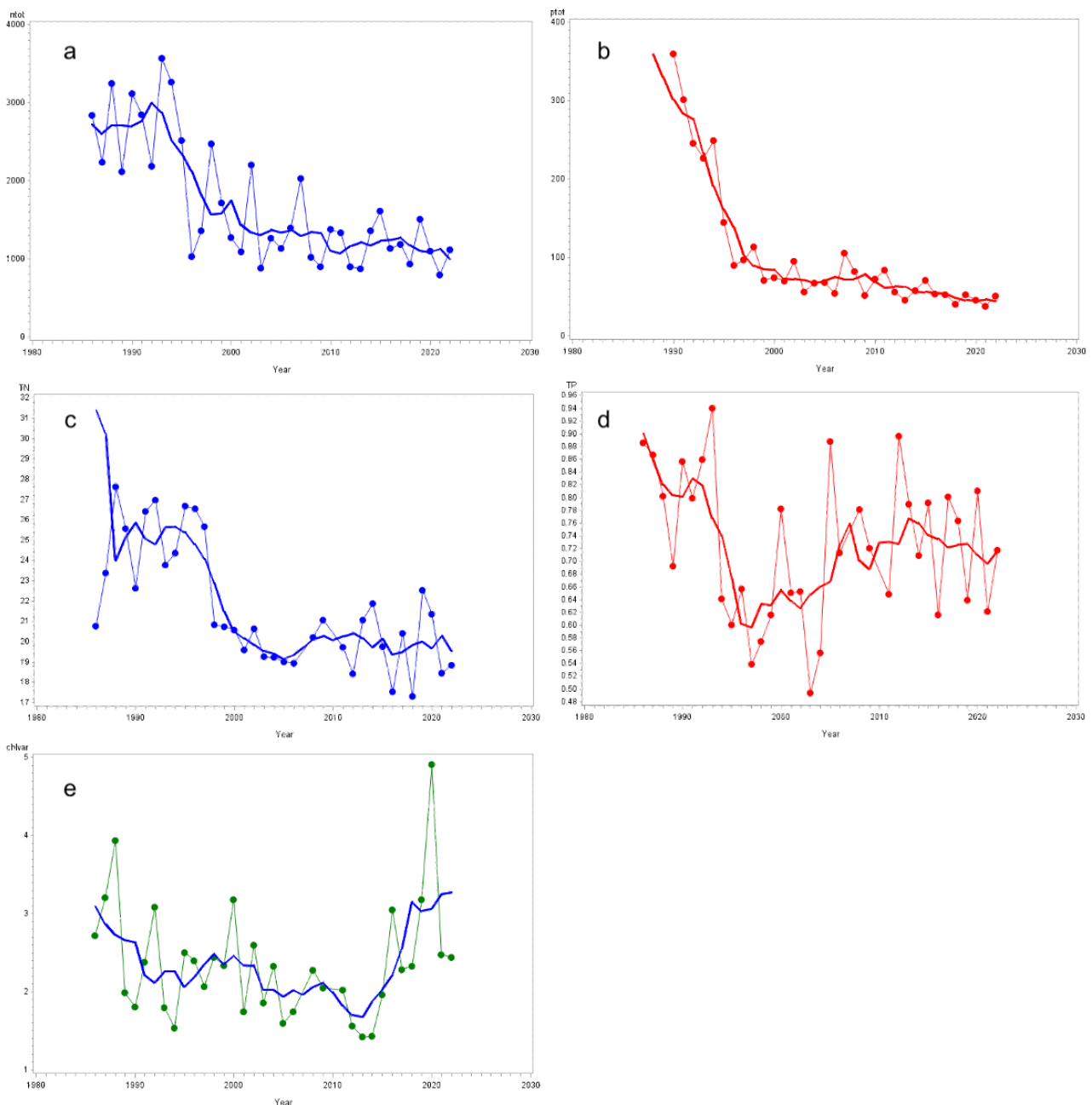
Figur 1.1. Tidlig udvikling i tilførsler af kvælstof i tons/år (a), fosfor tons/år (b) og koncentrationer af total kvælstof i µmol/l (c), total fosfor µmol/l (d) og klorofyl µg/l (e) for NOVANA station 1722 i Køge Bugt. Den markerede linje repræsenterer et 5 års glidende gennemsnit.
