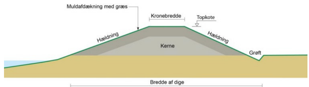
Figur 4-1: Principtegning af et kystdige (Kystdirektoratet, 2018)
