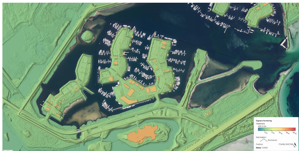
Figur 9-10: 3D præsentation af indre og ydre dige med sikringsniveau 320 cm DVR90 langs Hundige Strand og Ishøj Strand i Ishøj Kommune
