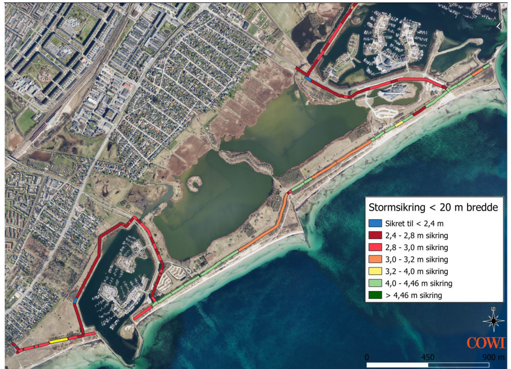
Figur 3-10: Højder for oversvømmelsesbeskyttelsen med en bredde på minimum 1 m og under 20 m, der definerer de ydre digers styrke. Vestlige del af Køge Bugt Strandpark
