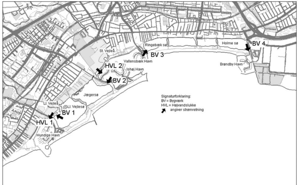
Figur 3-19 Højvandslukker (HVL) og bygværker (BV) i Køge Bugt Strandpark. De 6 slusebygværker leder dels bagvand fra Li. Vejle Å ud via HVL 1 og fra St. Vejleå ud via HVL 2 samt bagvand fra fæstningskanalen/Vestvolden ud via BV 4. Resten håndterer lagunerens vandudskiftning, se også Figur 3-15.
